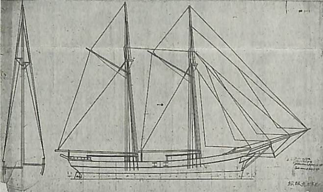
①伊勢市の有形文化財に指定された「旧市川造船所資料」に含まれる「松坂丸」装帆図 ②同時に指定された「朝熊町の河崎音頭」 ＝いずれも伊勢市教育委員会提供
