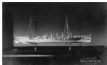
MNCL 1912 平戸 川崎造船 1911.6.29.進水
