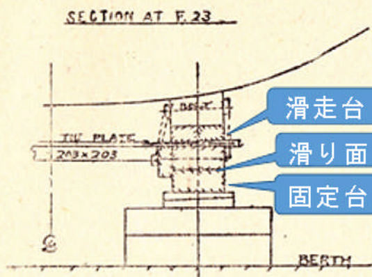
船体後部の進水台の断面図
