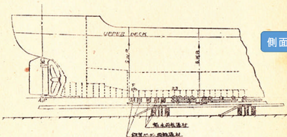
船体後部の進水台の断面図
