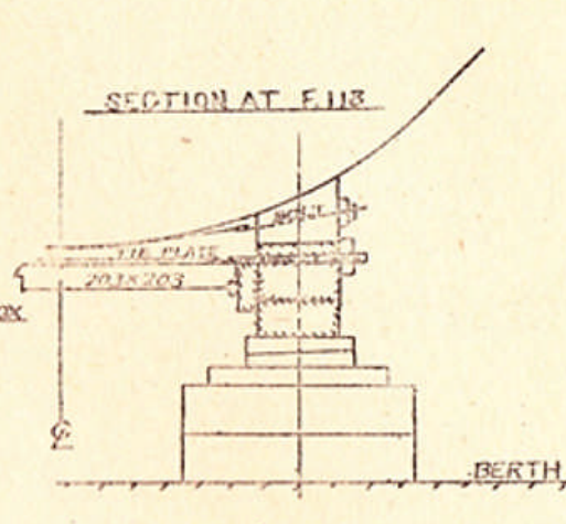
船体前部の進水台
